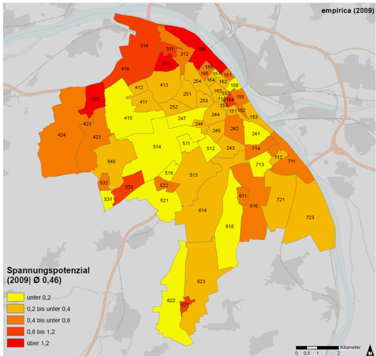
Karte 25: Spannungspotential
