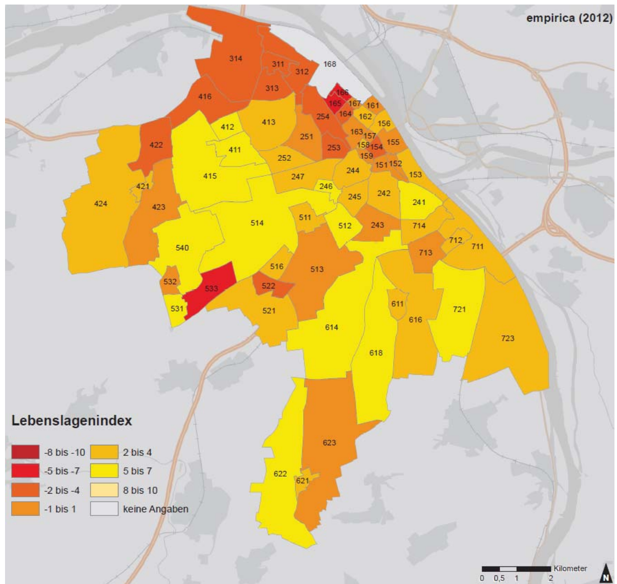
Karte 78: Lebenslagenindex
